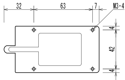
流速センサ裏面ネジ穴寸法 (面速式流量センサ固定用)
